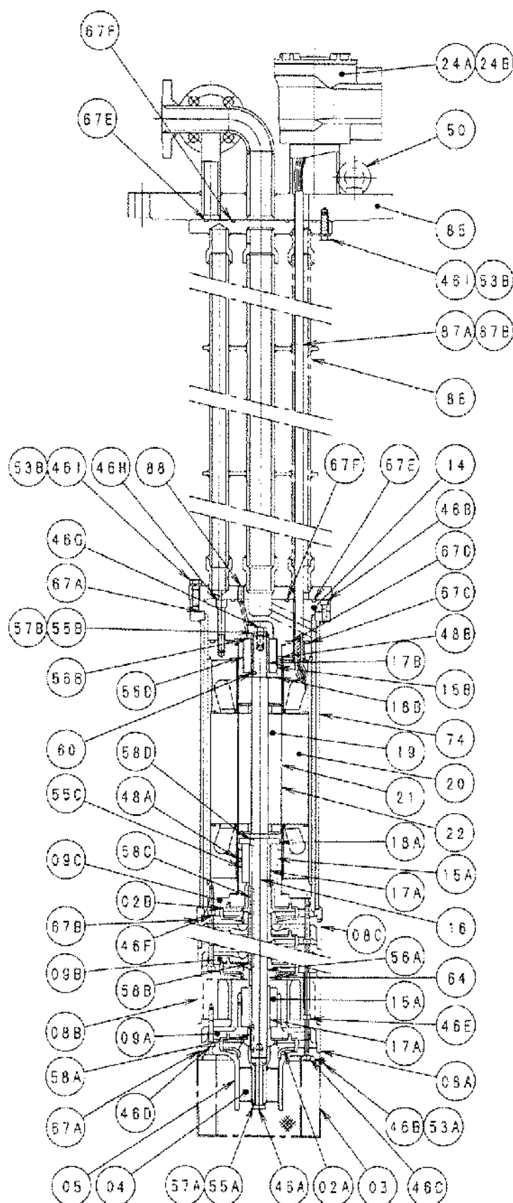
図1 構造断面図
